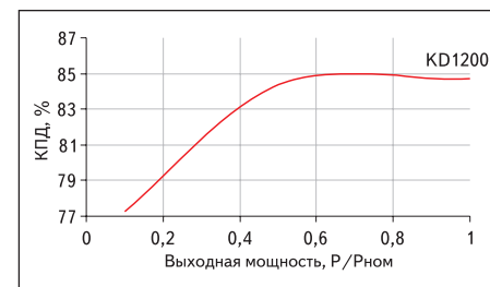
Рис. 4. График зависимости КПД модуля питания серии «Кедр» от нагрузки
