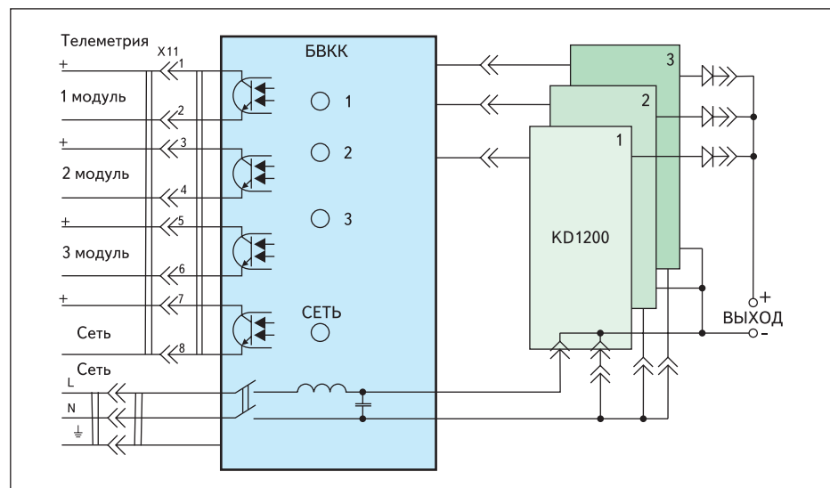
Рис. 8. Структурная схема модульного выпрямителя ВУ-3000
