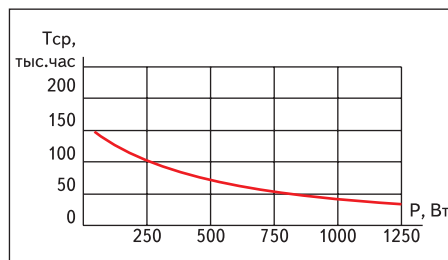
Рис. 1. График зависимости времени наработки на отказ от выходной мощности преобразователя
