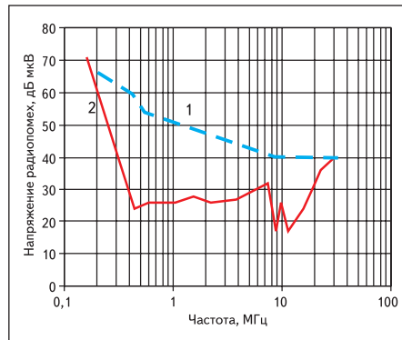
Рис. 6. Графики напряжения радиопомех: 1 — кривая «2» Норм по ГОСТ В 25803-91, 2 — уровень помех на входе модуля питания серии «Кедр»
