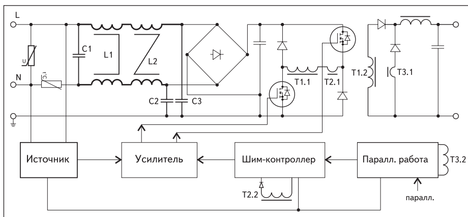
Рис. 5. Структурная схема модуля питания серии «Кедр»
