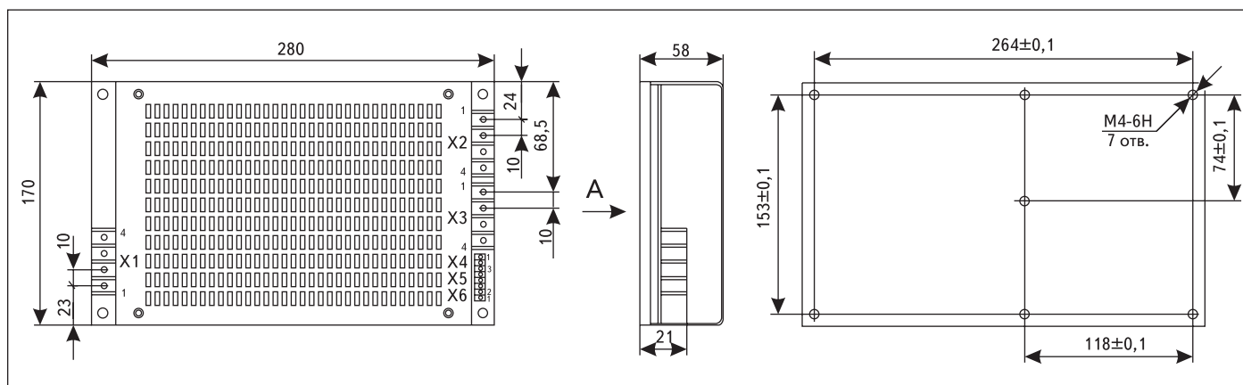
Рис. 3. Габаритные чертежи модуля питания серии «Кедр»
